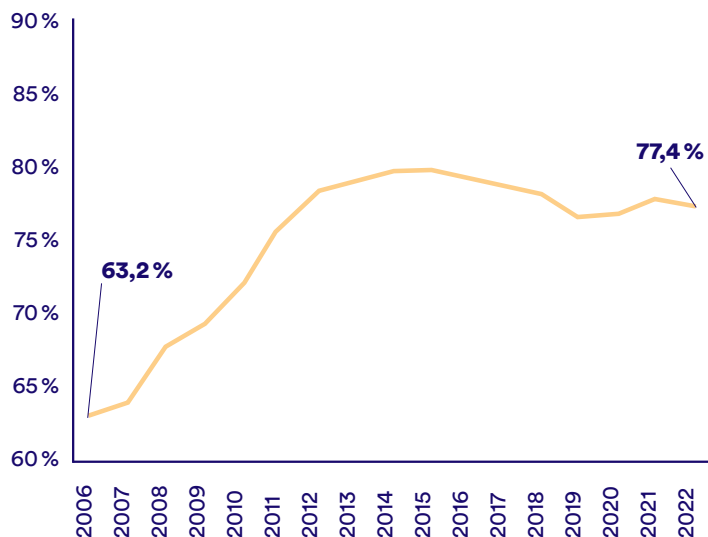
FIGURE 3. ÉVOLUTION DE LA PART DES CHAUSSÉES EN BON ÉTAT
